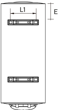
Instalación Vertical
